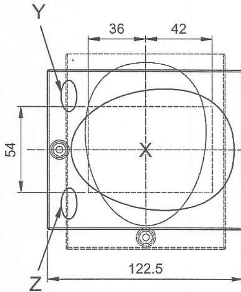
Ansicht von Vorne/front view
