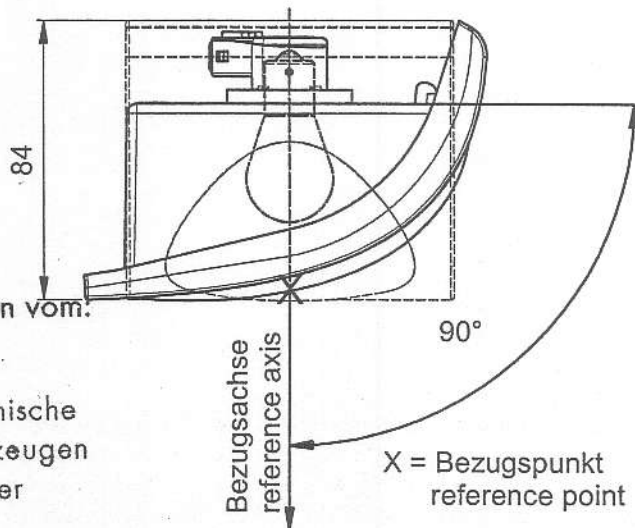
Ansicht von Oben/top view
