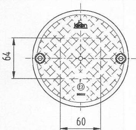
VUE DE FACE / Ansicht von Vorne / front view
