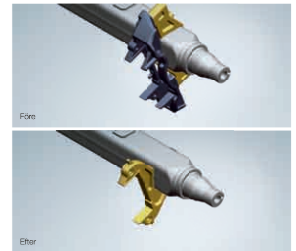
Jämförelse före-efter: Bromsen är för första gången direkt monterad på axelkroppen genom Compact Design.
