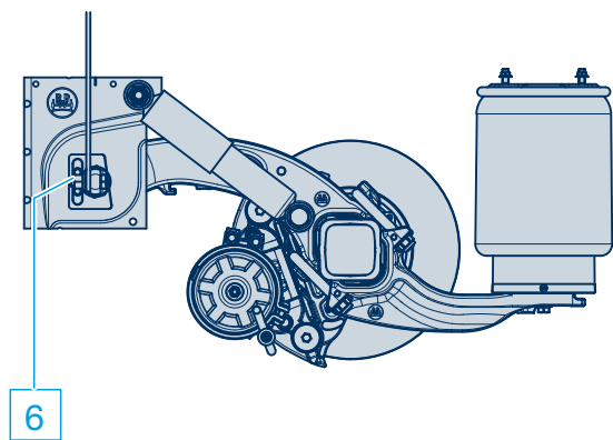
Typ ACBM med skruvbar knutplåt
