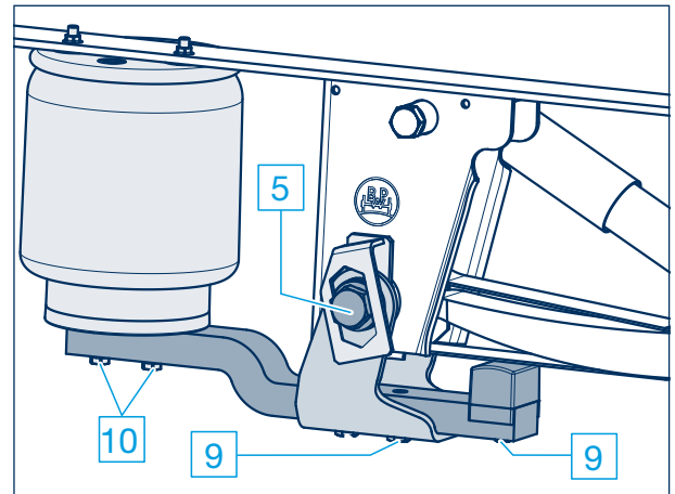
Sidomonterad lyft
