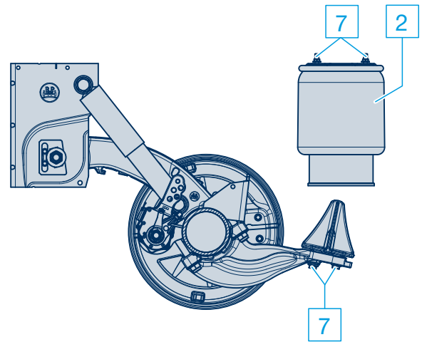
Typ EABO med Kombi-Air Bag II
