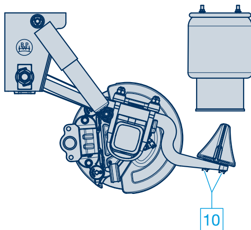
Typ ALM/SLM med Kombi-Air Bag II
