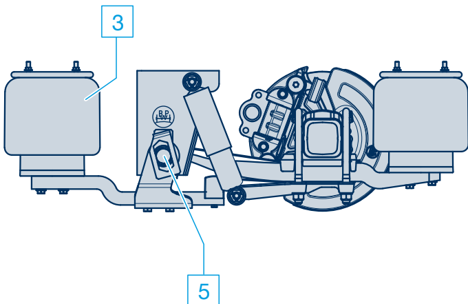
Typ ALU/SLU med sidomonterad axellyft
