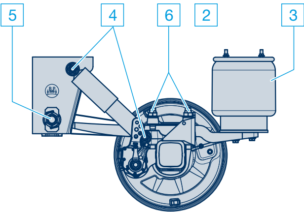
Typ ALO/SLO
