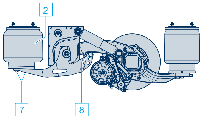
Typ ACAM med sidomonterad axellyft
