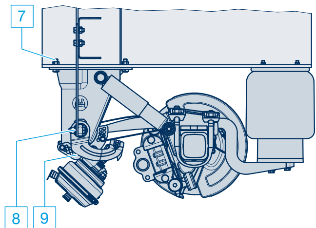
Typ ALM/SLM med skruvbart främre fäste och tvåsides axellyft
