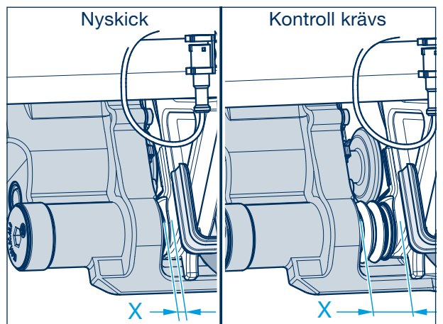
Skivbroms typ TSB
