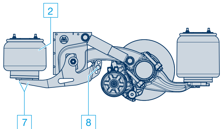
Typ EAAM med sidomonterad axellyft
