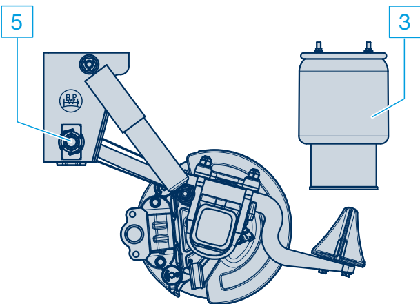
Typ ALM/SLM med Kombi-Air Bag II
